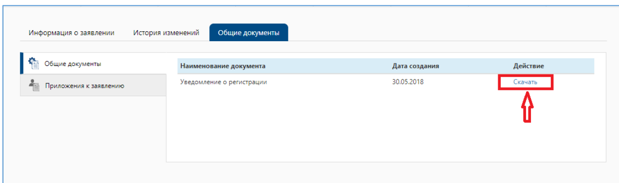
Рисунок 13. Выходные документы
