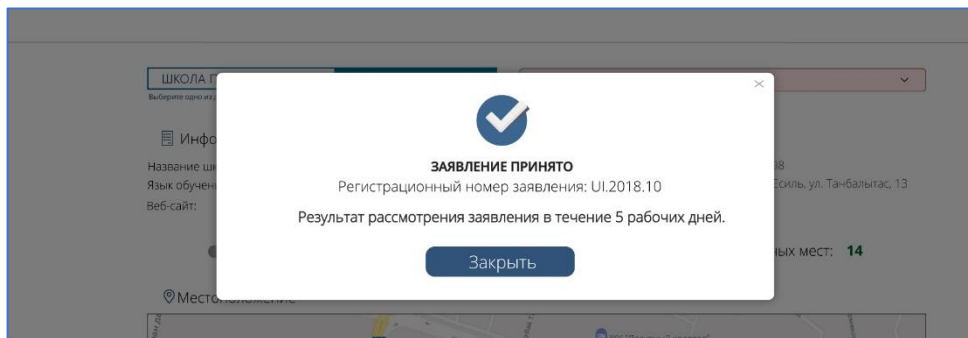
Рисунок 10. Уведомительное окно
